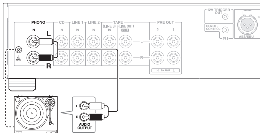
Проигрыватель грампластинок (MM) без встроенного усилителя-корректора.
