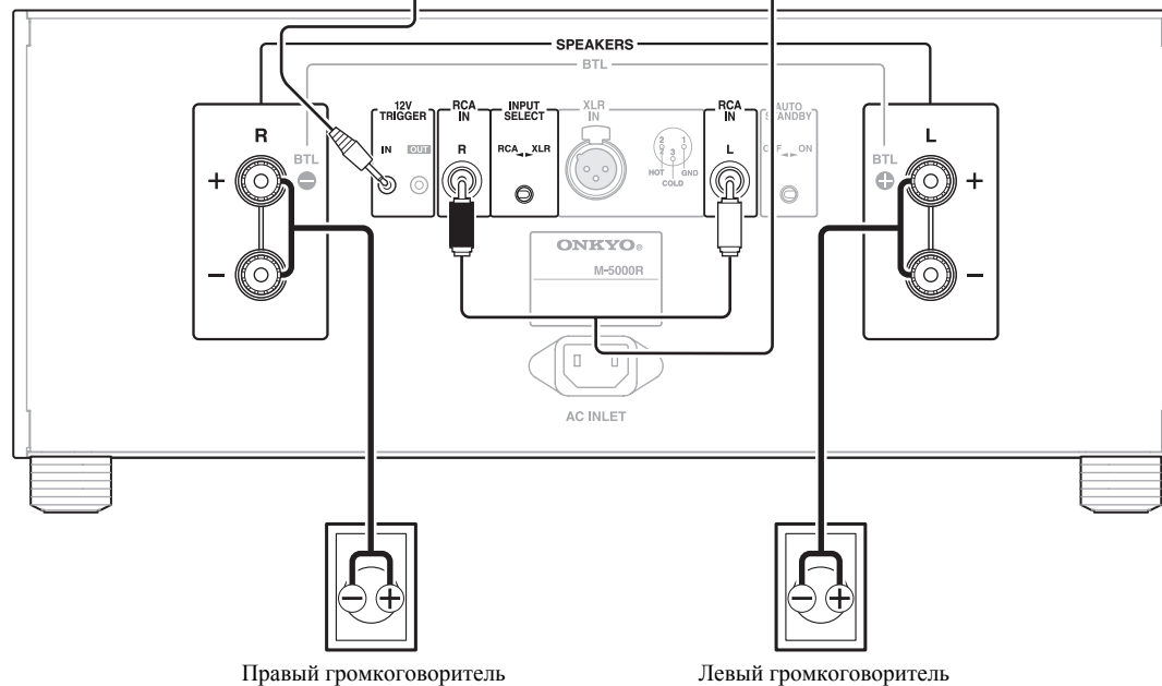
Это – пример стерефонического соединения, использующего усилитель мощности M-5000R.
